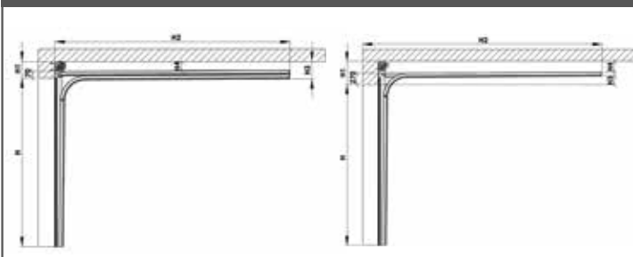
Dintel Alto - HL | Dintel Vertical - VL
