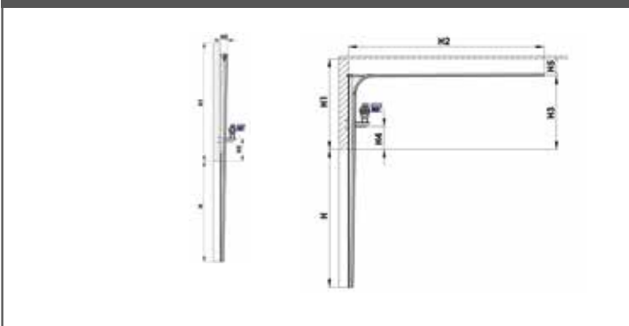
Dintel Vertical - VAL | Dintel Alto - AL
